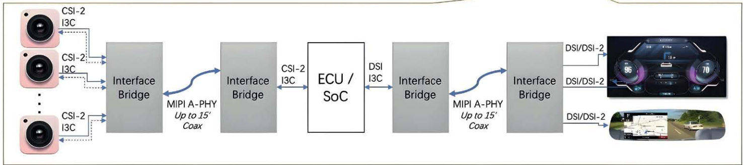
Bild 2: FPGAs können als intelligente Schnittstelle zwischen anderen Komponenten eingesetzt werden, die unterschiedliche Schnittstellenstandards oder -protokolle verwenden.
