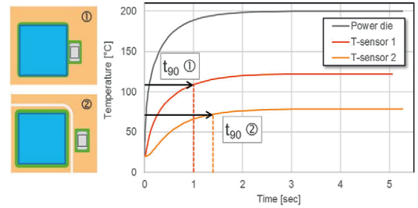
Bild 5: Temperaturverhalten beim Einschalten des Power-Die. Temperatursensor 1 befindet sich in der Nähe des Power-Die, Temperatursensor 2 ist durch einen geätzten Graben vom Power-Die getrennt.
