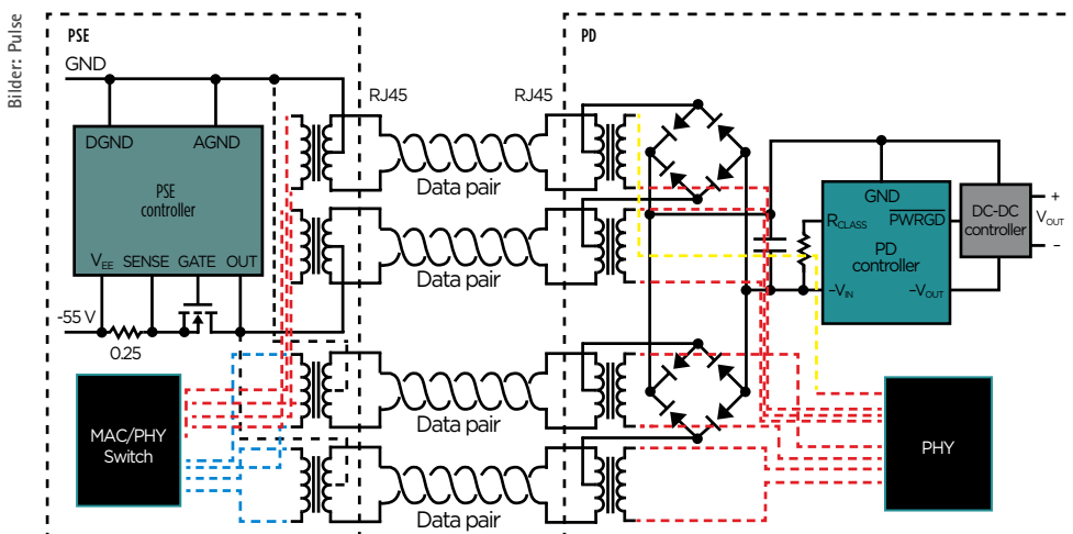
Bild 1: Funktionsweise von PoE
